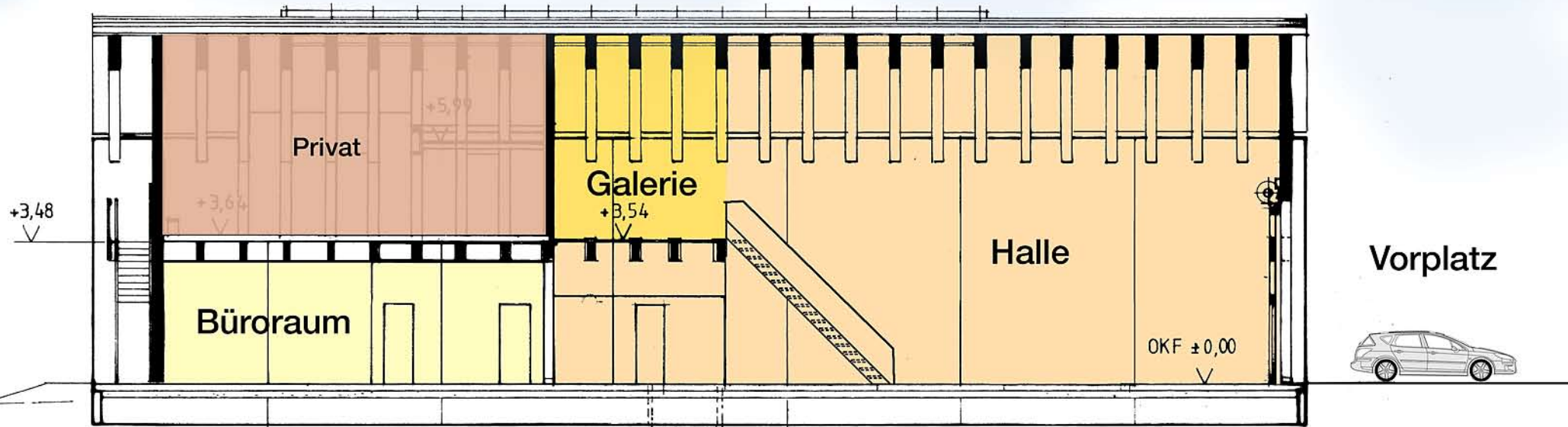
LÄNGSSCHNITT
